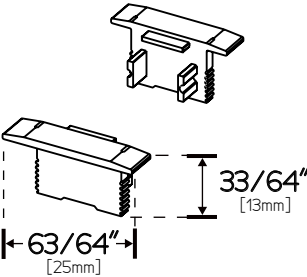
LE2513-EC End Cap
